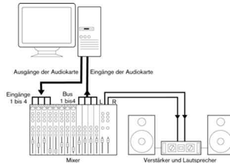
Ein Mehrkanal-Audioaufbau mit externem Mischpult.
