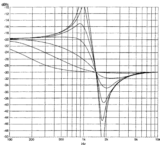
MPX 1 Parametric EQ: Shelf
