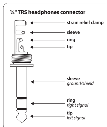
Rys. 4.2: Stereofoniczny wtyk typu Jack 6,3 mm
