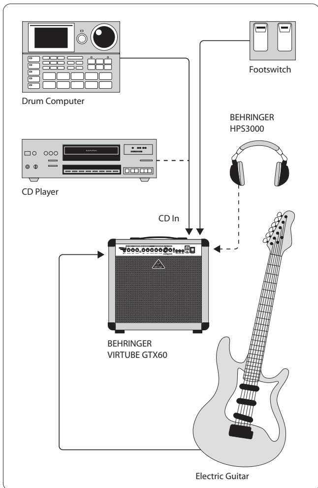
Rys. 3.1: Standardowa konfiguracja urządzenia GTX60
