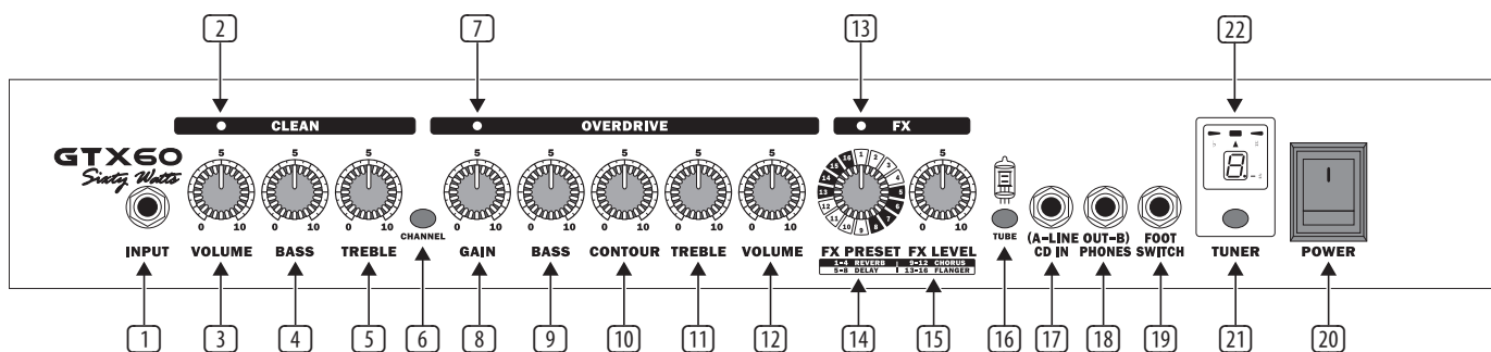
Rys. 2.1: Elementy obsługi GUITAR COMBO (płyta czołowa)
